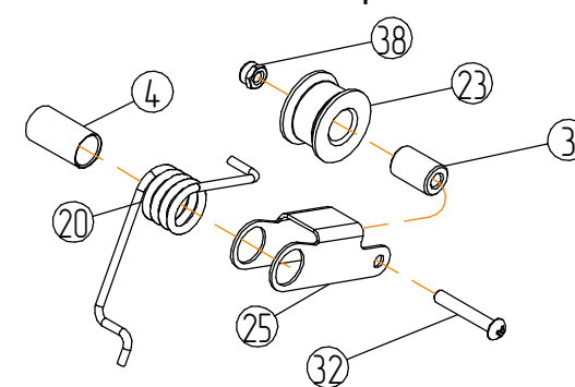
Натяжитель цепи
