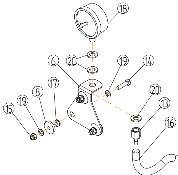
Виброопора тягомера
