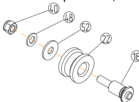
Ролик направляющий
