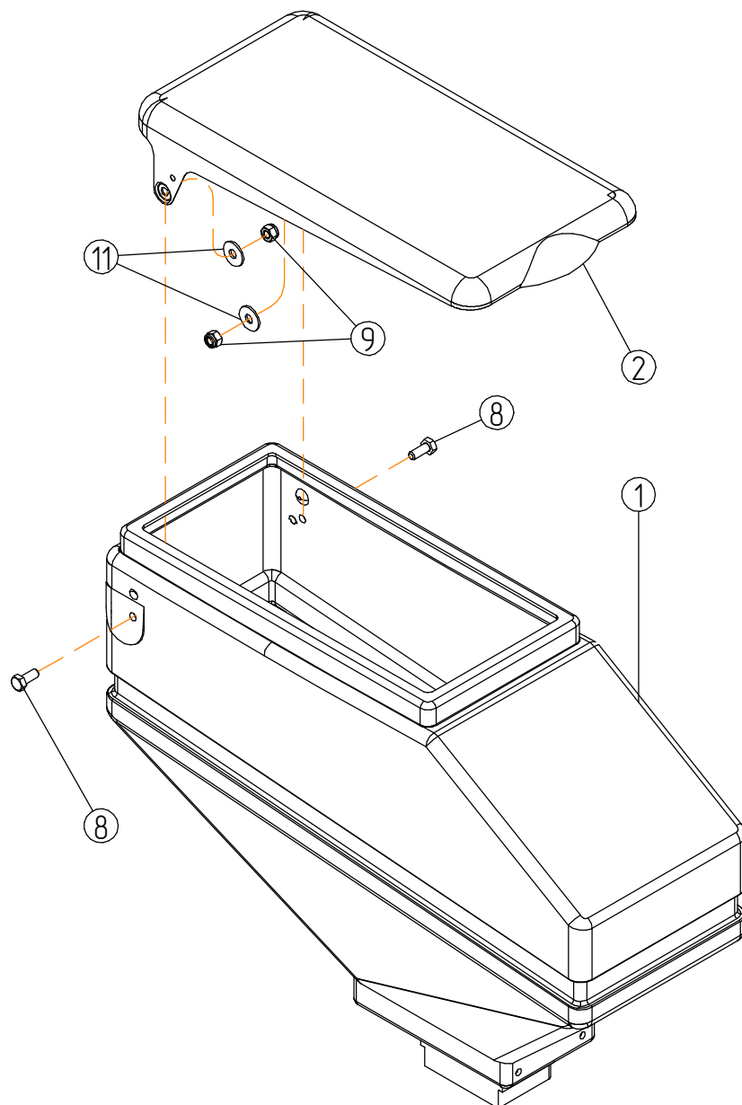
Бункер семян
